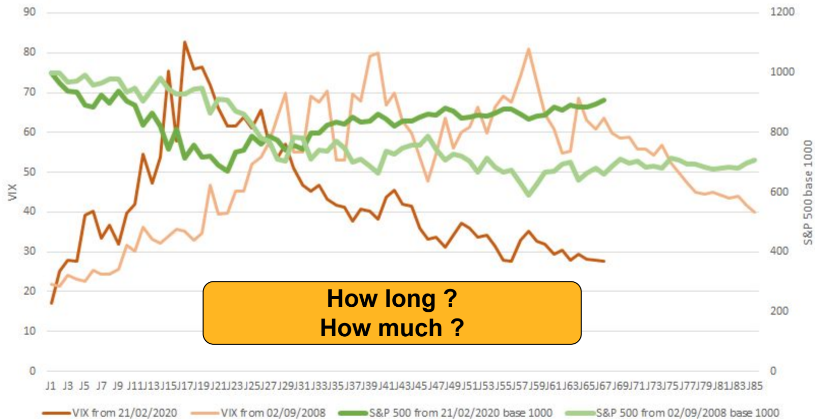
VIX & S&P 500 index
